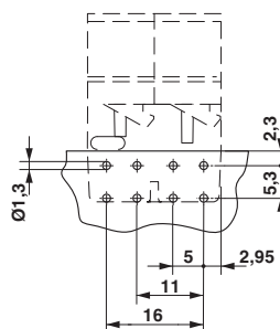
Vrtací schéma
