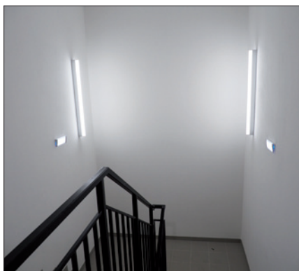
Obr. 2. Všechny prostory jsou vybaveny nouzovým a antipanickým osvětlením
